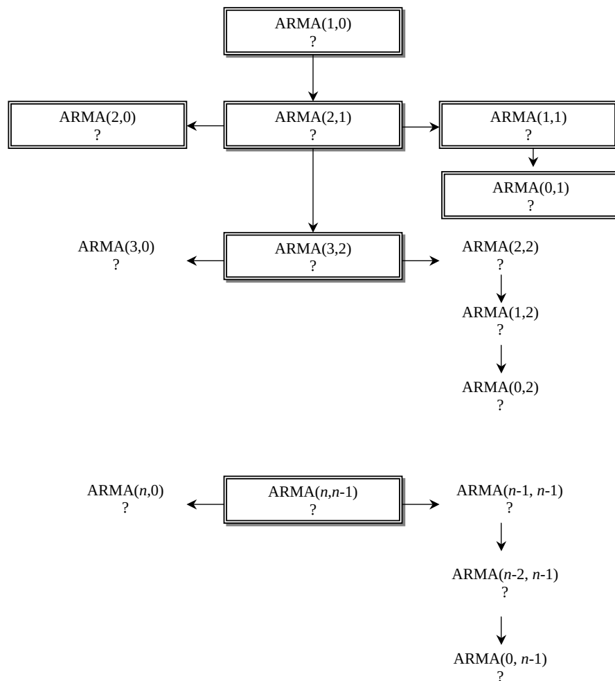
Рис. 15. Процесс выбора ARIMA модели
